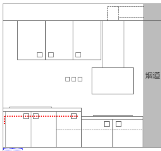
橱柜侧视图：
